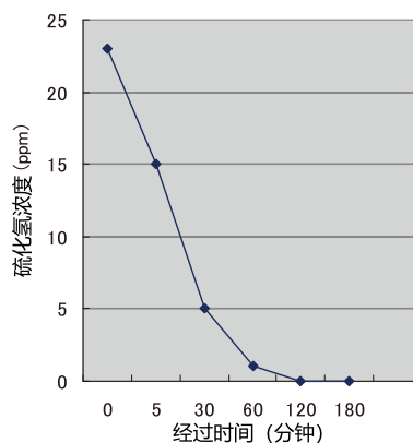
硫化氢（腐败臭味）的浓度降解试验
